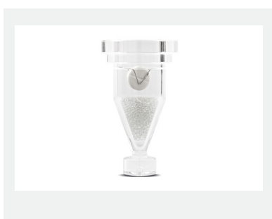
CELDA PARA COMPRIMIDOS (22,6 MM) CON MICROESFERAS DE VIDRIO (1)
